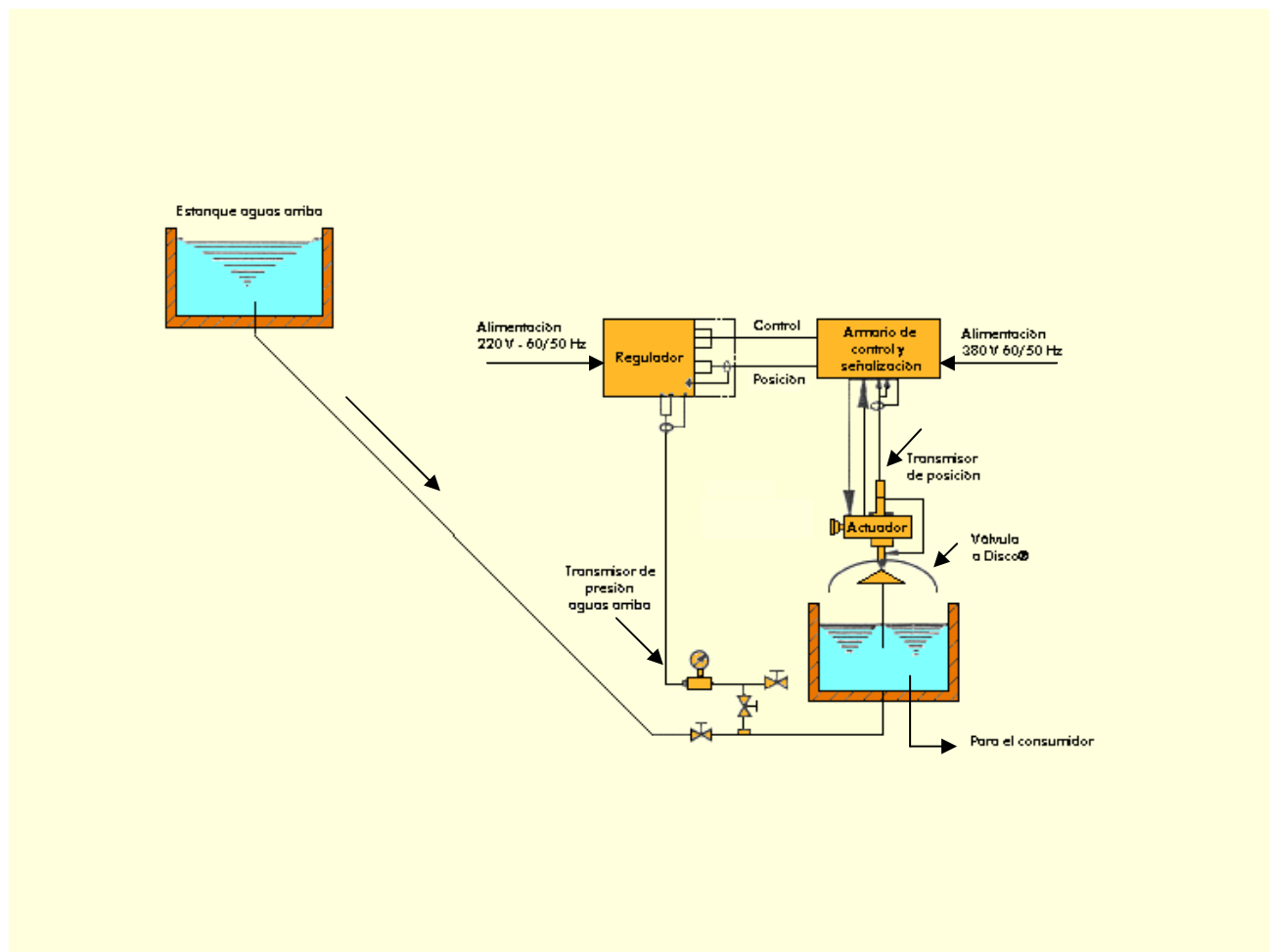
Esquema de regulación de caudal
